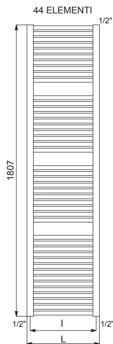
Particolare della versione con 2 manicotti laterali (vedi pagine seguenti)
