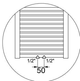
Particolare della versione interasse 50 mm.
